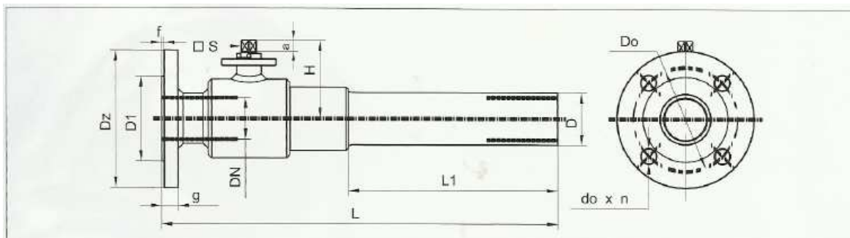
Wymiary podstawowe
